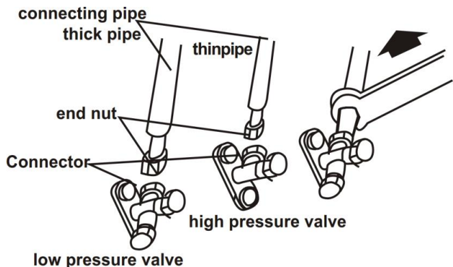
Obrázek 3. 5 Potrubí a schéma zapojení zařízení
