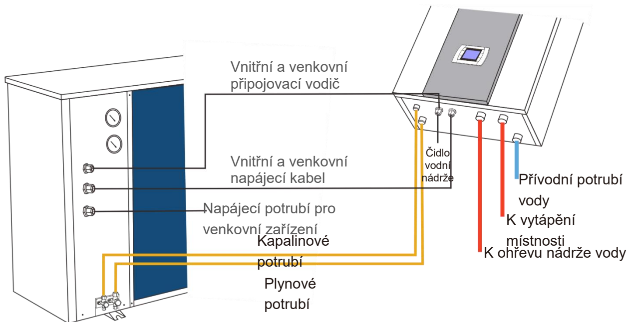
Obrázek 3. 5 Potrubí a schéma zapojení zařízení
